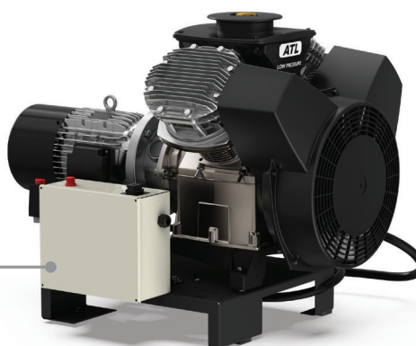
ATL-4-BTX 4 kW, na základovém rámu
